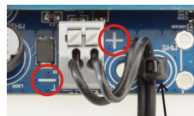
Bild 9: Steckernetzteil am Mainboard anschließen
